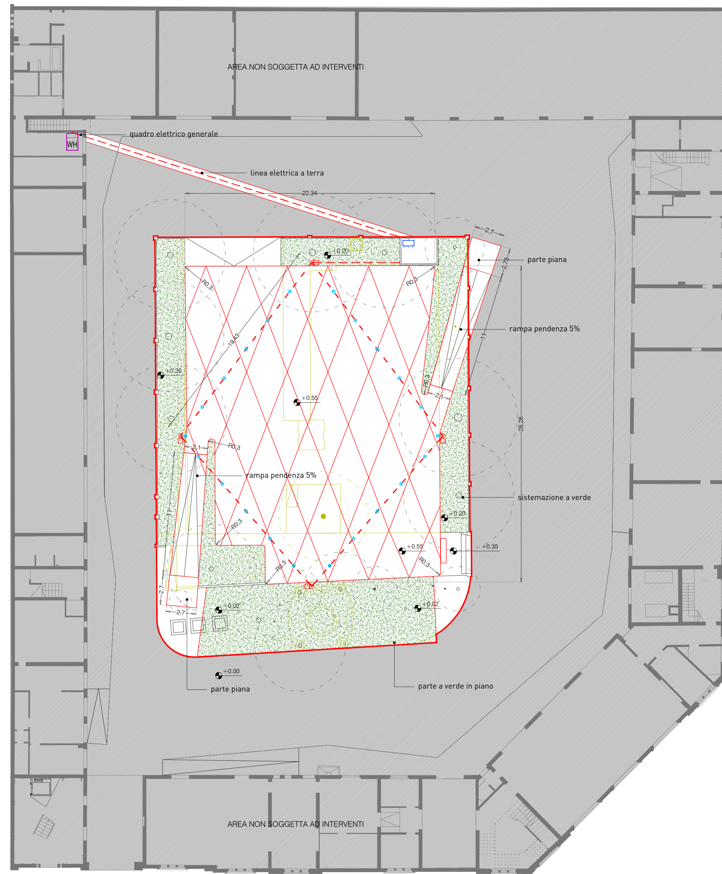
demolizioni e costruzioni - 1:200
